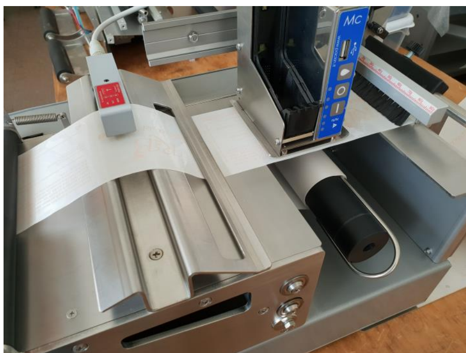
Pk-52 con marcatore inkjet modello Mc e fotocellula per etichette trasparenti (Leuze ad ultrasuoni).
